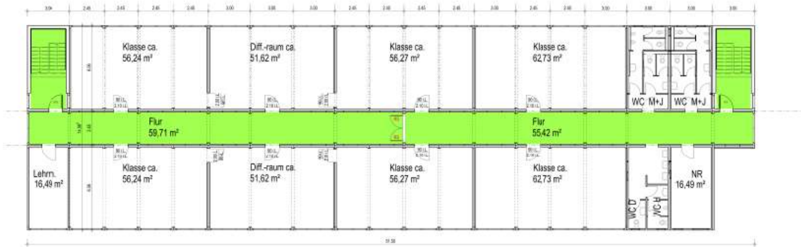
Obergeschoss Ausbaustufe 1
